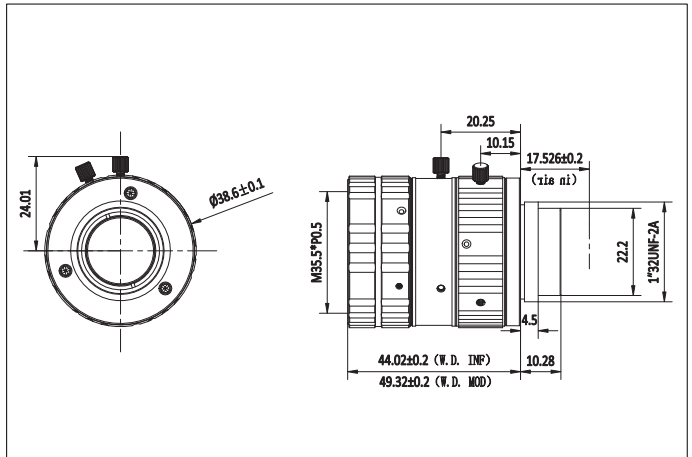
尺寸图
