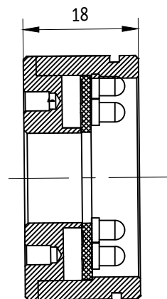
剖视图 B-B
