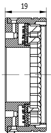
剖视图 A-A
