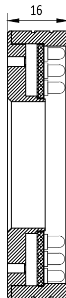
剖视图 A-A
