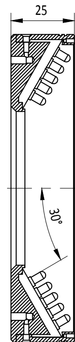
剖视图 A-A
