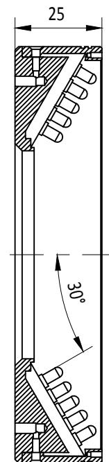
剖视图 A-A
