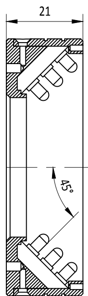
剖视图 A-A
