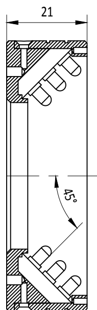
剖视图 A-A
