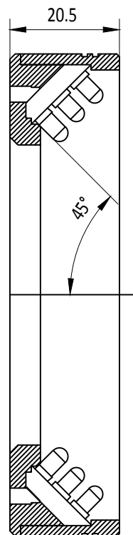
剖视图 A-A
