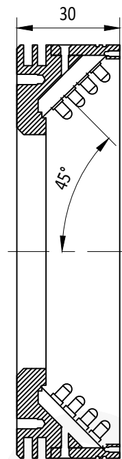
剖视图 A-A
