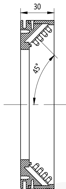
剖视图 A-A
