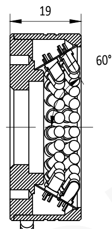
剖视图 A-A
