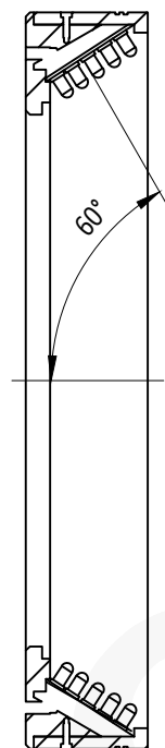
剖视图 A-A
